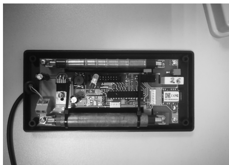
Фиг. 5: "Гайгерови броячи"
